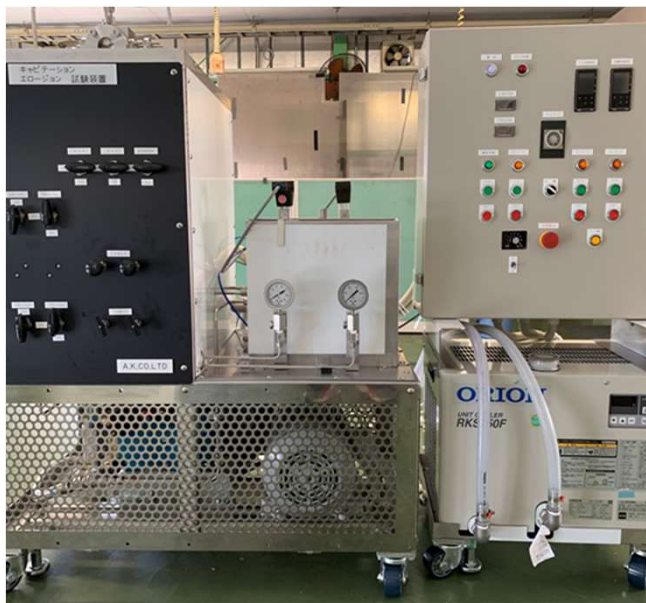
キャビテーション噴流試験装置
